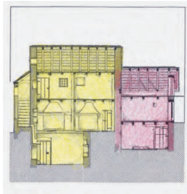
Schnitt durch zwei der translozierten Wohnhäuser. Gelb: das sogenannte Doppelhaus von ca. 1865. Rot: das sogenannte Eckhaus von ca. 1741.
